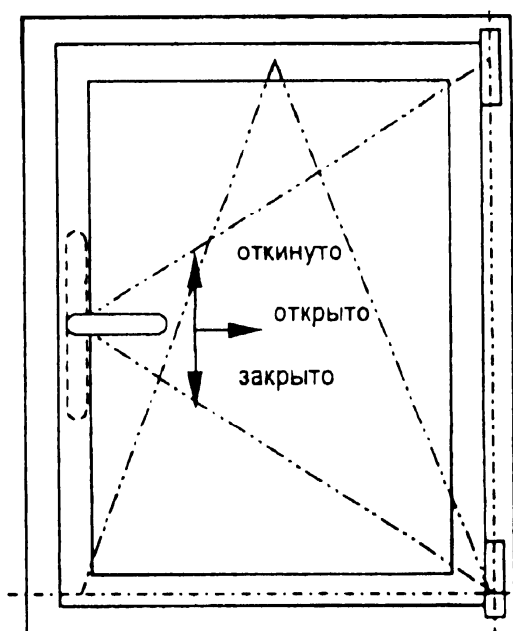
Рисунок А.3 - Устройство поворотно-откидное
