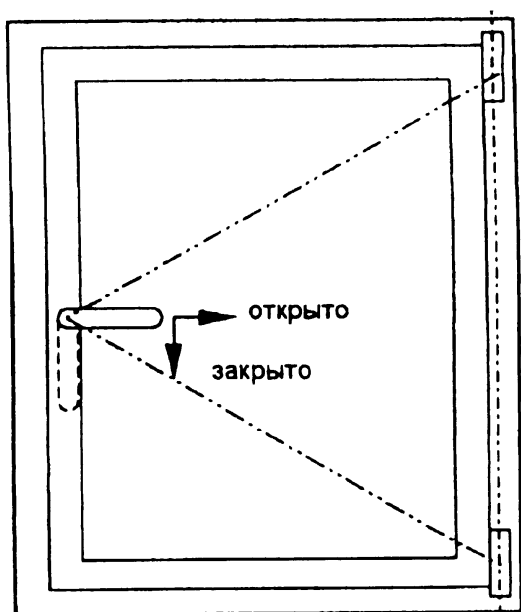
Рисунок А.1 – Устройство поворотное
