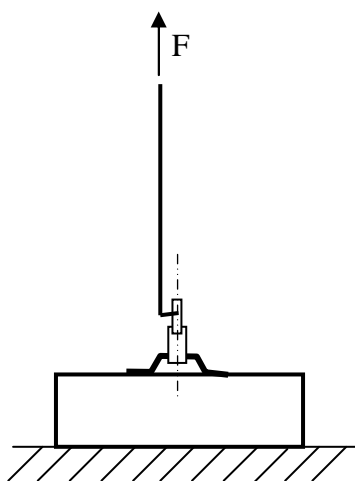
Рисунок В.1 - Схема приложения статической нагрузки на верхнюю петлю
