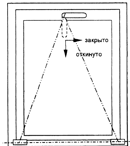
Рисунок А.2 – Устройство откидное
